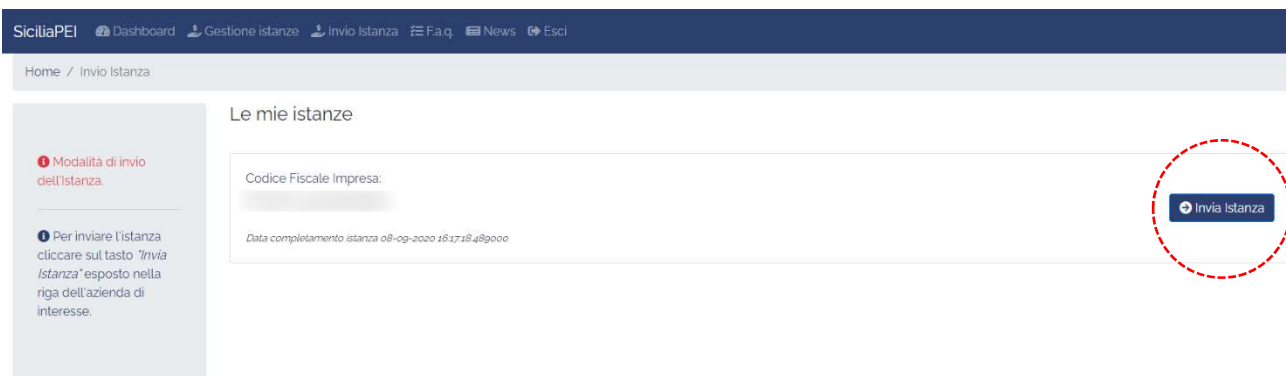
Figura 23 - Invio Istanza
